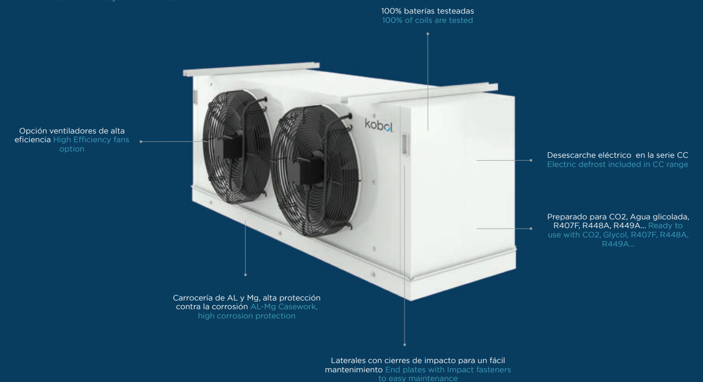
Laterales con cierres de impacto para un fácil mantenimiento End plates with Impact fasteners to easy maintenance
