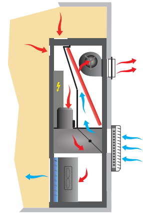
RAFFREDDAMENTO COOLING
